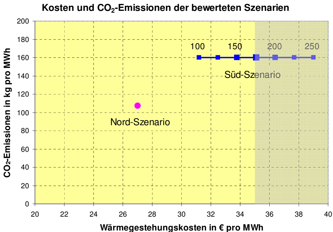
Bild 12: Gegenüberstellung von Wärmegegestehungskosten und CO 2 -Emissionen des Nord-Szenarios und des Süd-Szenarios. Beim Süd-Szenario sind die Kosten für den Bau der Süd-Trasse in Mio. € als Parameter angegeben. 35 €/pro MWh ist nach [Sandrock 16, Seite 43] die Grenze für die Infragestellung der Wettbewerbfähigkeit bei den Wärmegegestehungskosten.
