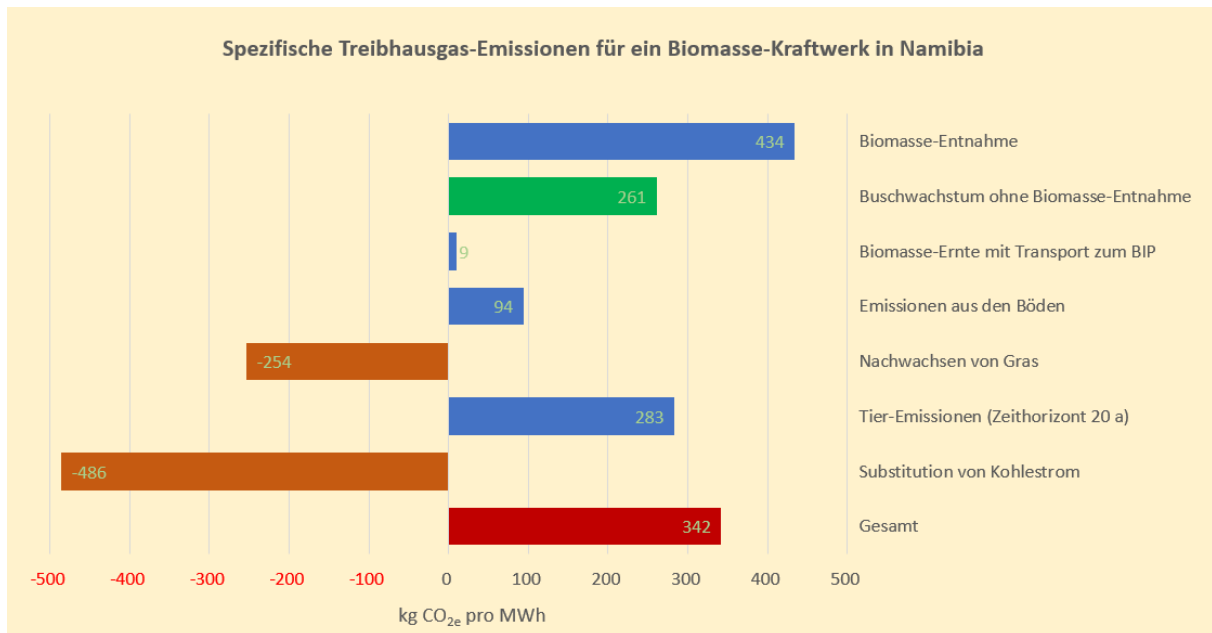
Bild 15: Treibhausgas-Bilanz für das Kraftwerks-Szenario 5 von [Seebauer 2019] nach Berücksichtigung von Parametern von NamPower und nach Durchführung von Korrekturen entsprechend Abschnitt 5.
